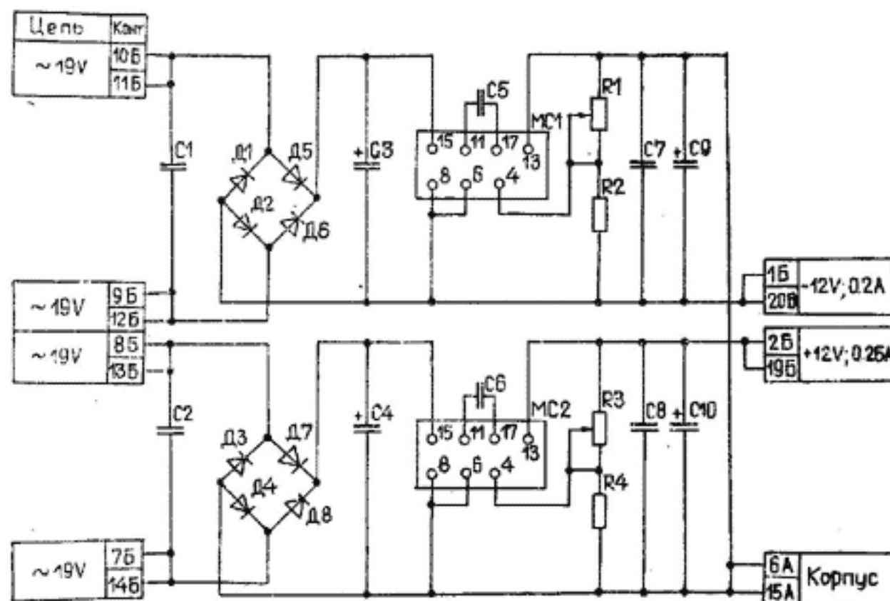
Блок стабилизаторов напряжения (3.233.063) Схема электрическая принципиальная.
