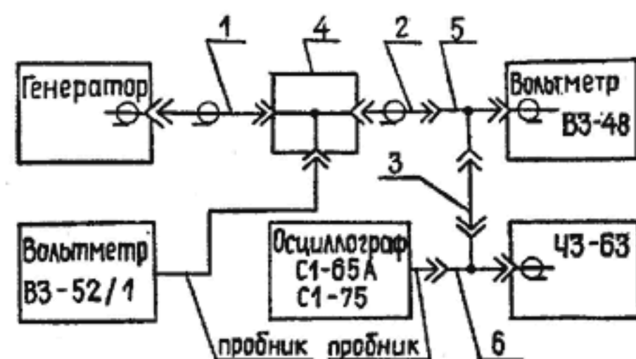
Структурная схема соединения приборов при проверке диапазона измеряемых частот
