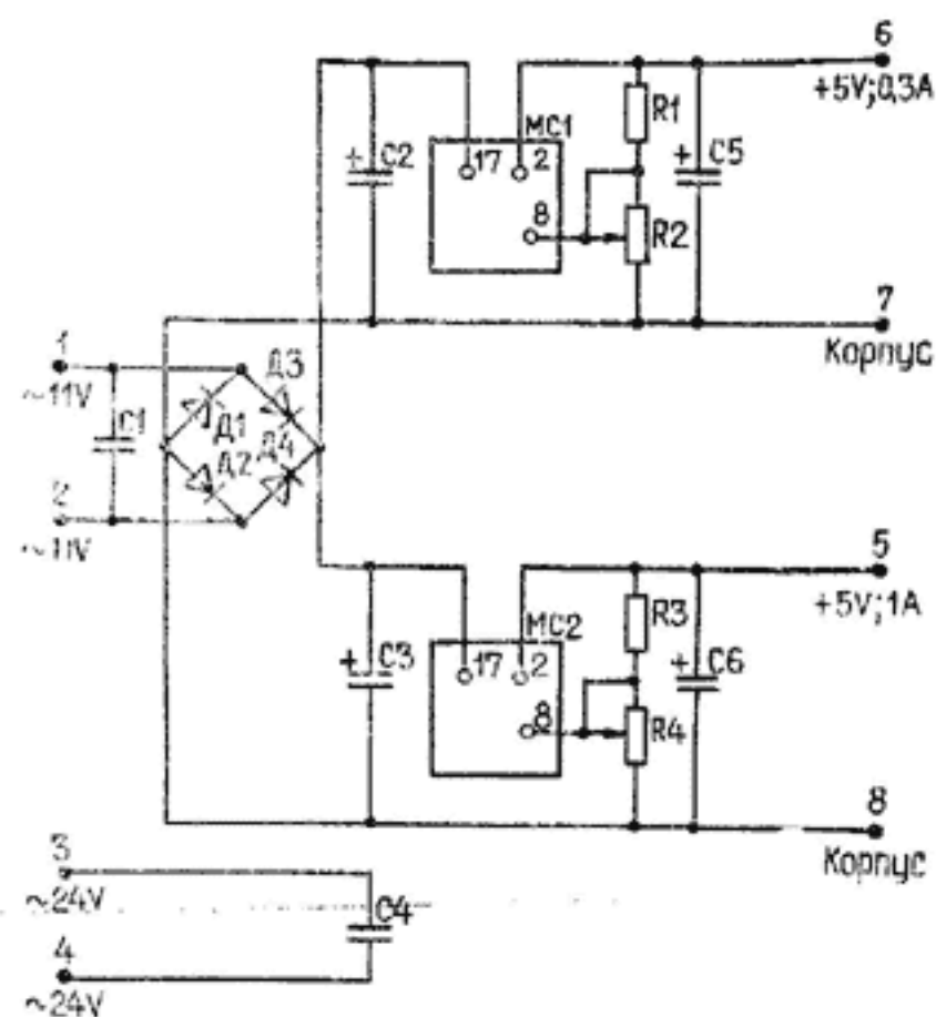
Блок стабилизаторов напряжения (3.233.099) Схема электрическая принципиальная.
