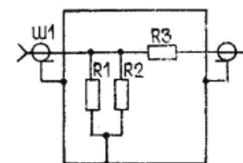
Аттенюатор (2.243.014) Схема электрическая принципиальная.
