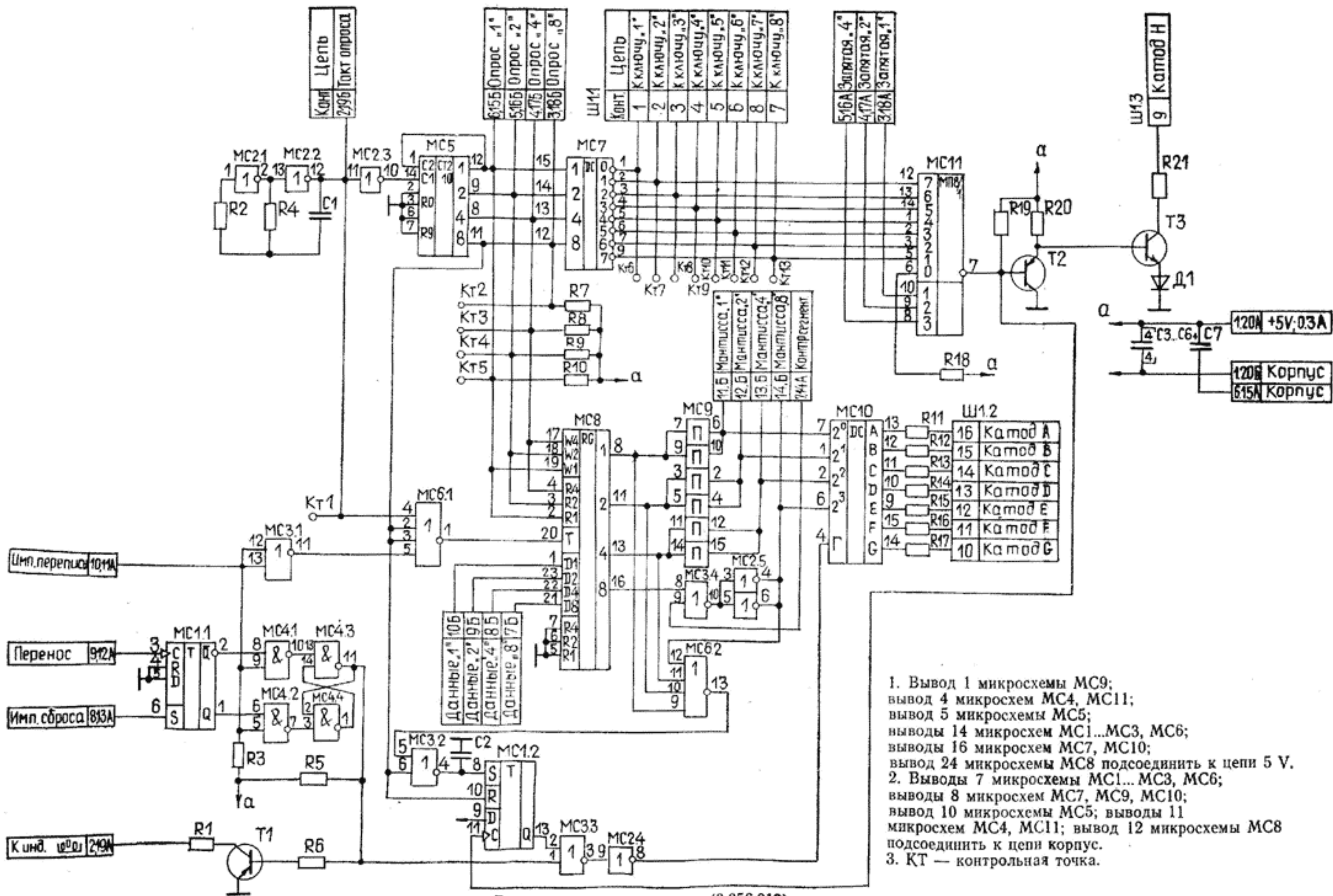
Распределитель импульсов (3.056.013). Схема электрическая принципиальная.
