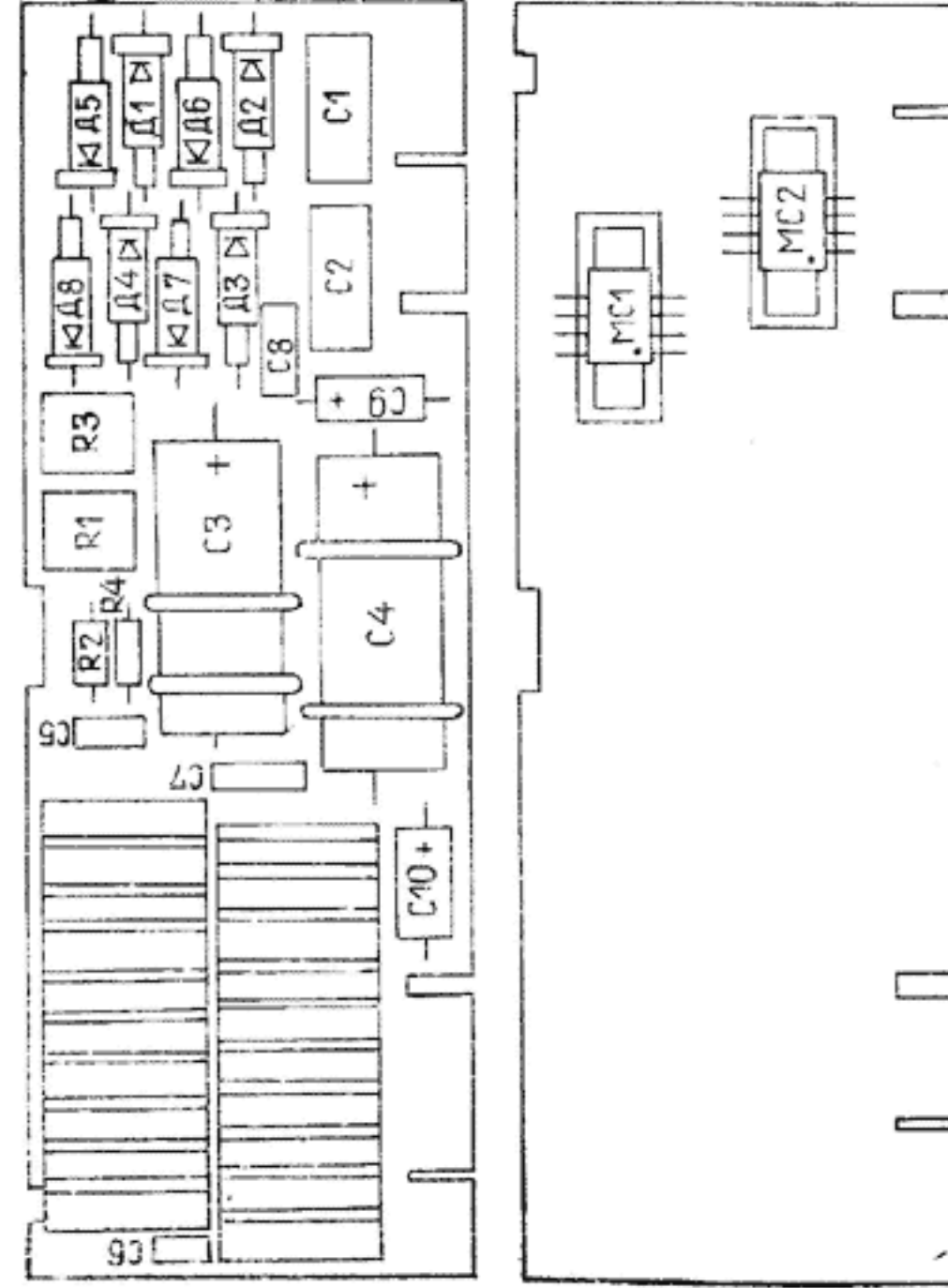
Блок стабилизаторов напряжения (3.233.063)
