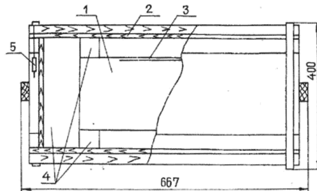
Схема упаковки
