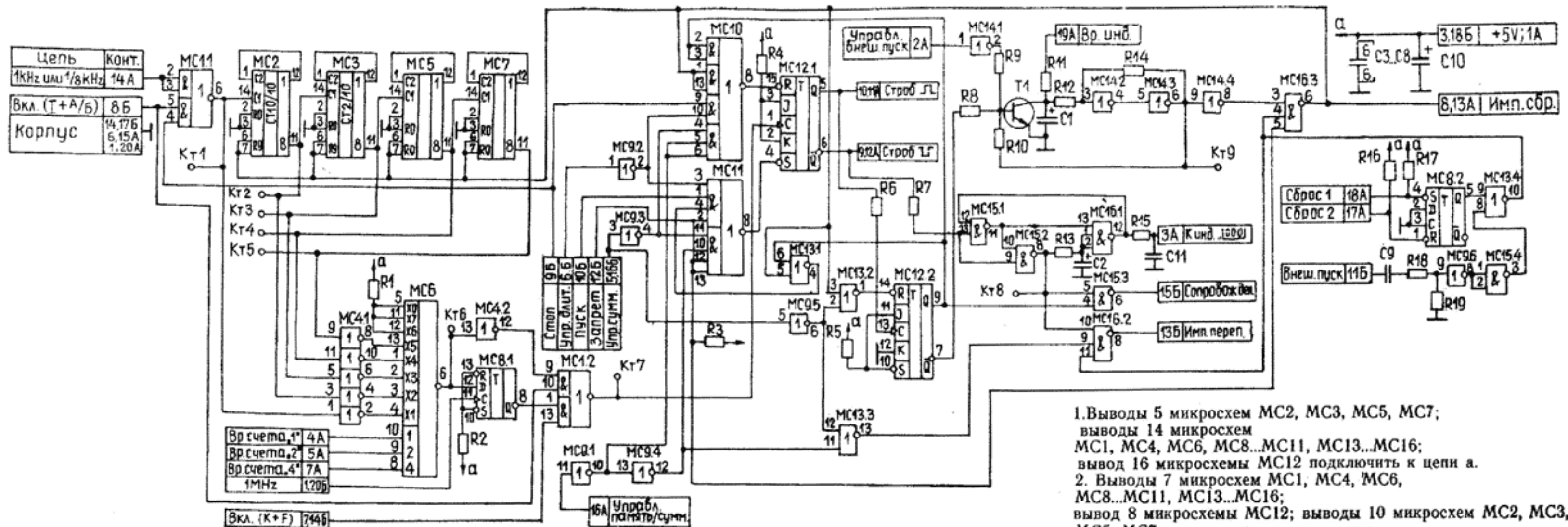
Блок автоматики (2.070.025) Схема электрическая принципиальная.
